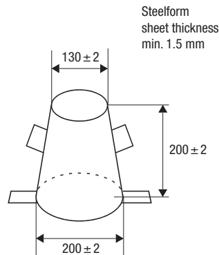
Fig. 5.2.6: Slump cone
