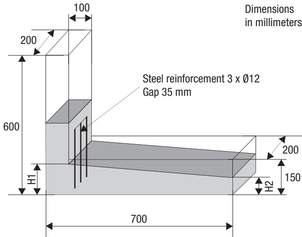
Fig. 5.2.8: L-Box test
